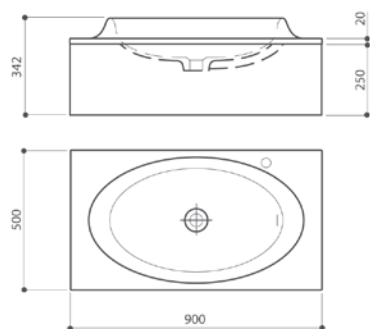
lavello 90x50 cm mobile con cassetto (versione unica) 90x50 cm basin with drawer (single version)
