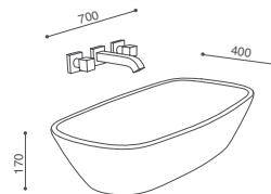
lavabo 70 cm d'appoggio 70 cm countertop basin
