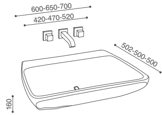
lavabo 60-65-70 cm d'appoggio 60-65-70 cm countertop basin
