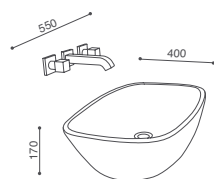
lavabo 55 cm d'appoggio 55 cm countertop basin
