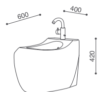
bidet sospeso wall-mounted bidet
